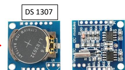
DS 1307
